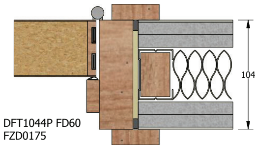
4-part Doorframe FD60
