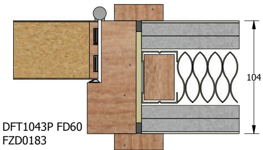
3-part Doorframe FD60
