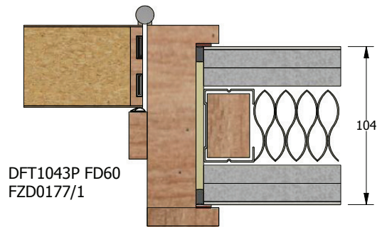
3-part Doorframe FD60
