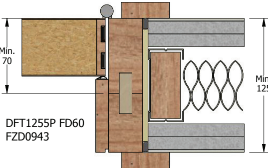
5-part Split Doorframe FD60
