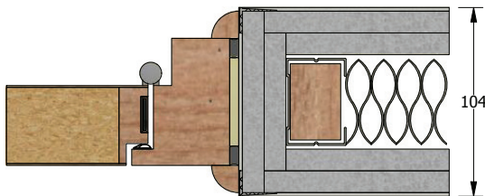
DFT701PR FD30 FZD0439
