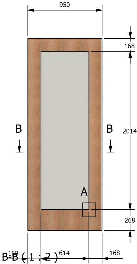
Front1 : 20 )
