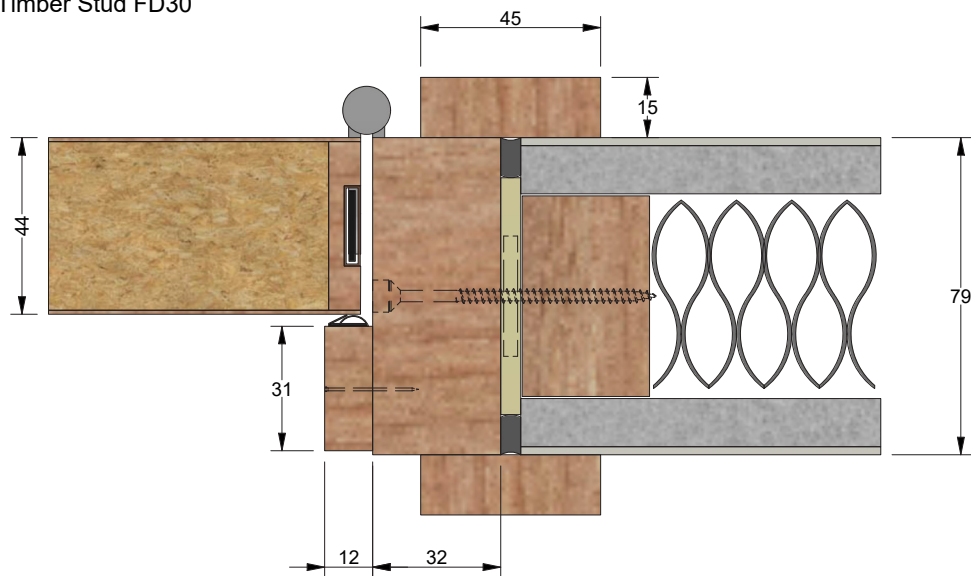
Dimensions Timber Stud FD30
