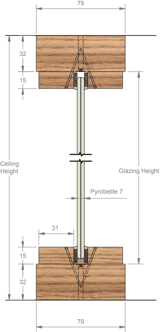
C-C (1:2)
