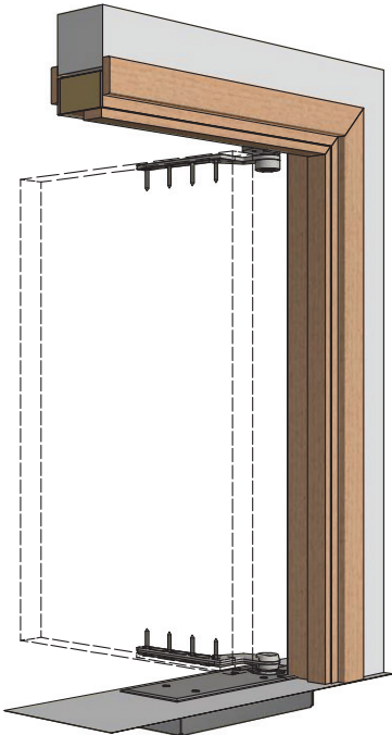
Perspective - door open
