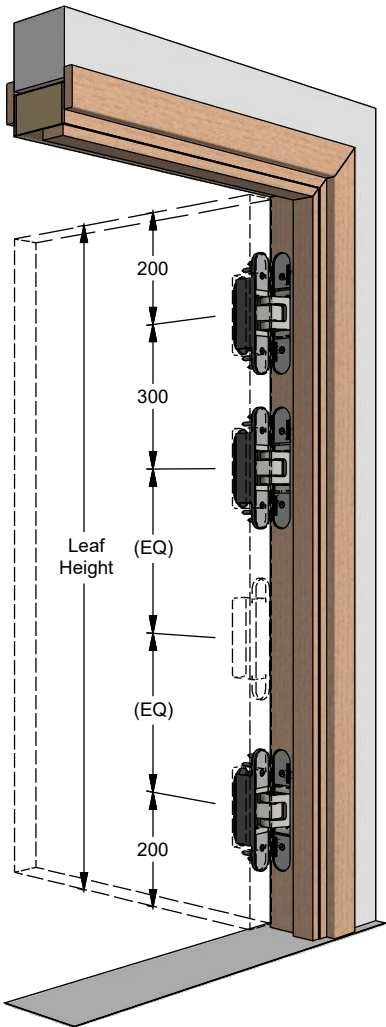
Perspective - door open
