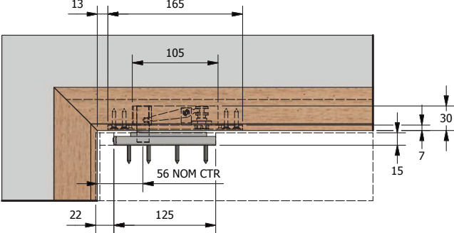
Door Head
