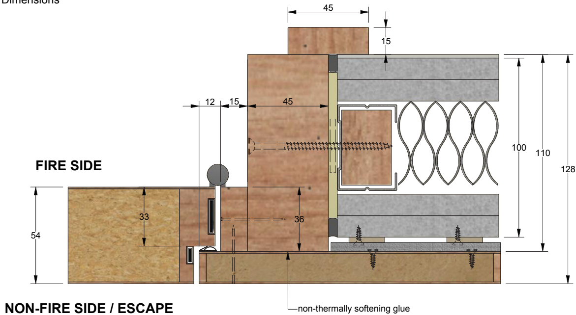
Dimensions
