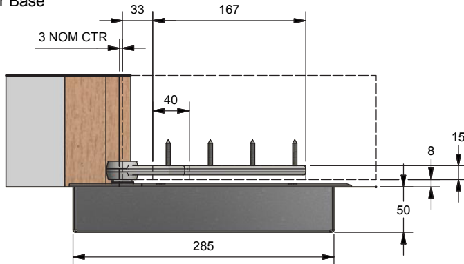
Door Base
