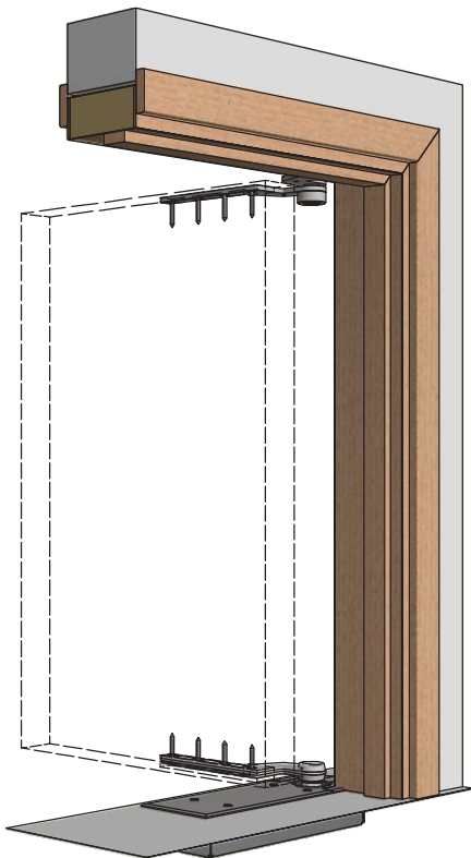
Perspective - door open
